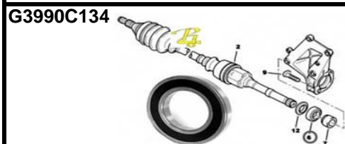
G3990C134 féltengely csapágy
