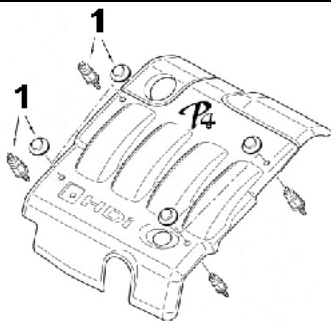
1. G0790A914 Hdi burkolattartó gumibak
